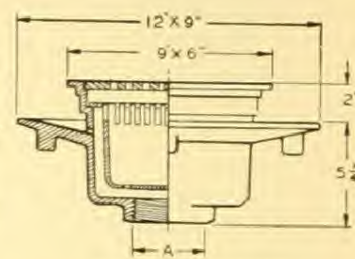
Z-585—I.P.S. Outlet
