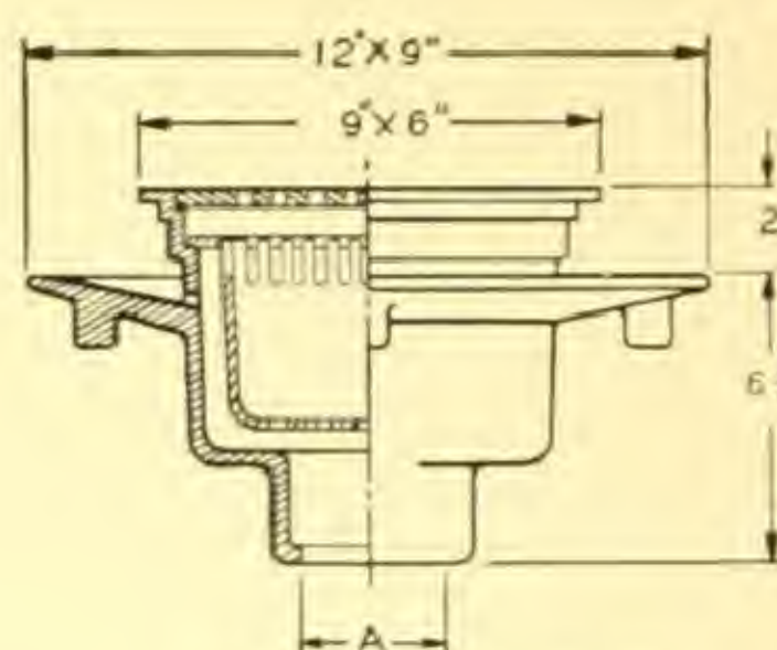
Z-585—Caulk Outlet
