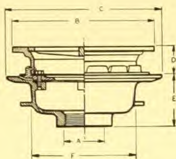
I.P.S. Outlet
