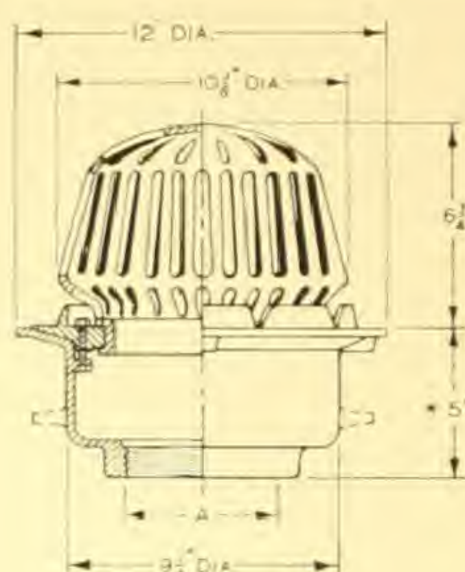
I.P.S. Outlet
